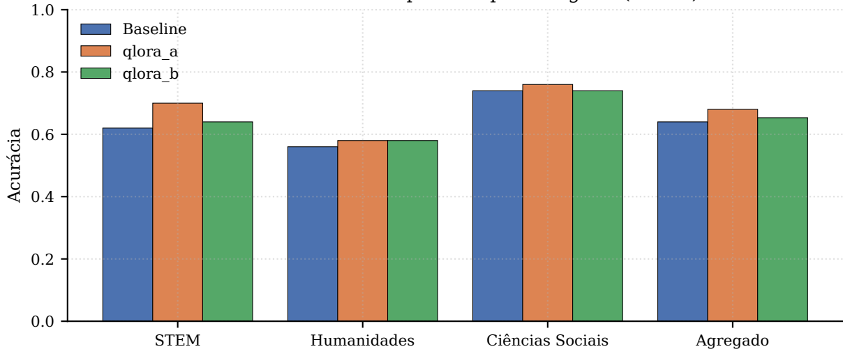
MMLU 5-shot — 50 questões por categoria (Fase 5)
