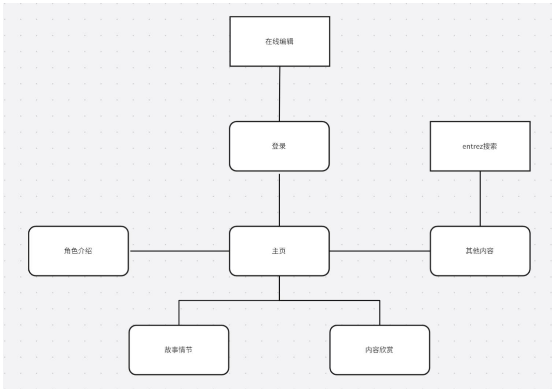
图 3-1 结构流程图
