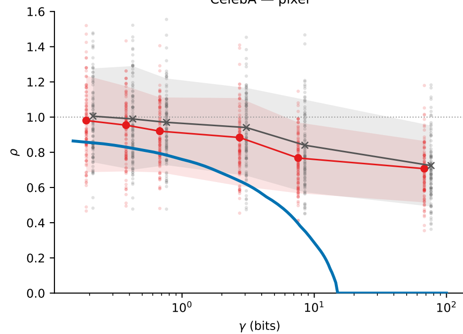
CelebA — pixel
