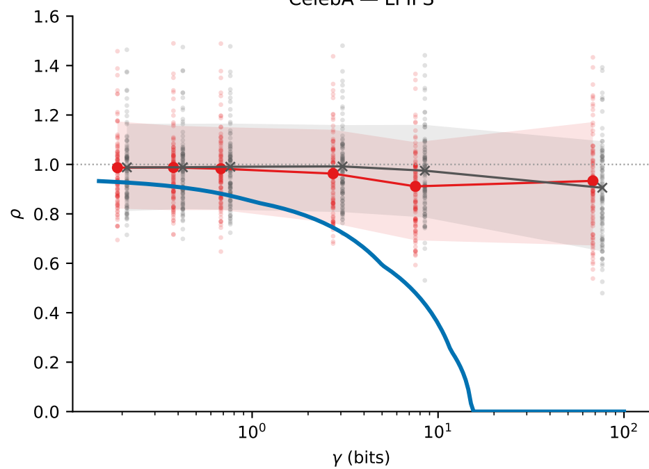
CelebA — LPIPS
