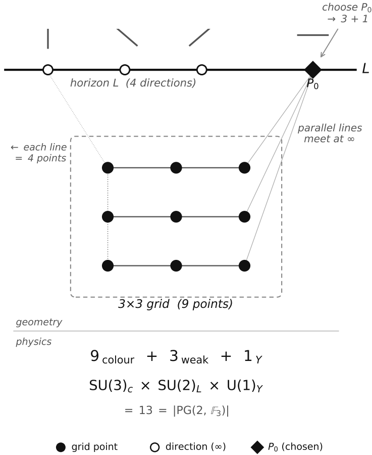
図 2. 射影平面 \text{PG}(2, \mathbb{F}_3) の構造。 3 \times 3 グリッド（9 点、黒丸）の平行線が無有限遠ライン L 上の方 向（白丸）で合流する。 P_0 （黒菱形）を選ぶことで 9+3+1 = 13 の分割が生じ、 \text{SU}(3) \times \text{SU}(2) \times \text{U}(1) のセクター構造に対応する。
