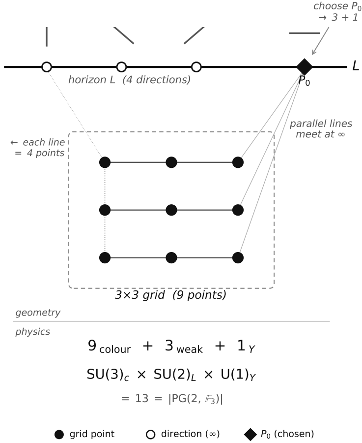
図2. 射影平面 \text{PG}(2, \mathbb{F}_3) の構造。3×3 グリッド（9点、黒丸）の平行線が無遠限ライン L 上の方角（白丸）で合流する。 P_0 （黒菱形）を選ぶことで 9+3+1=13 の分割が生じ、 SU(3) \times SU(2) \times U(1) のセクター構造に対応する。
