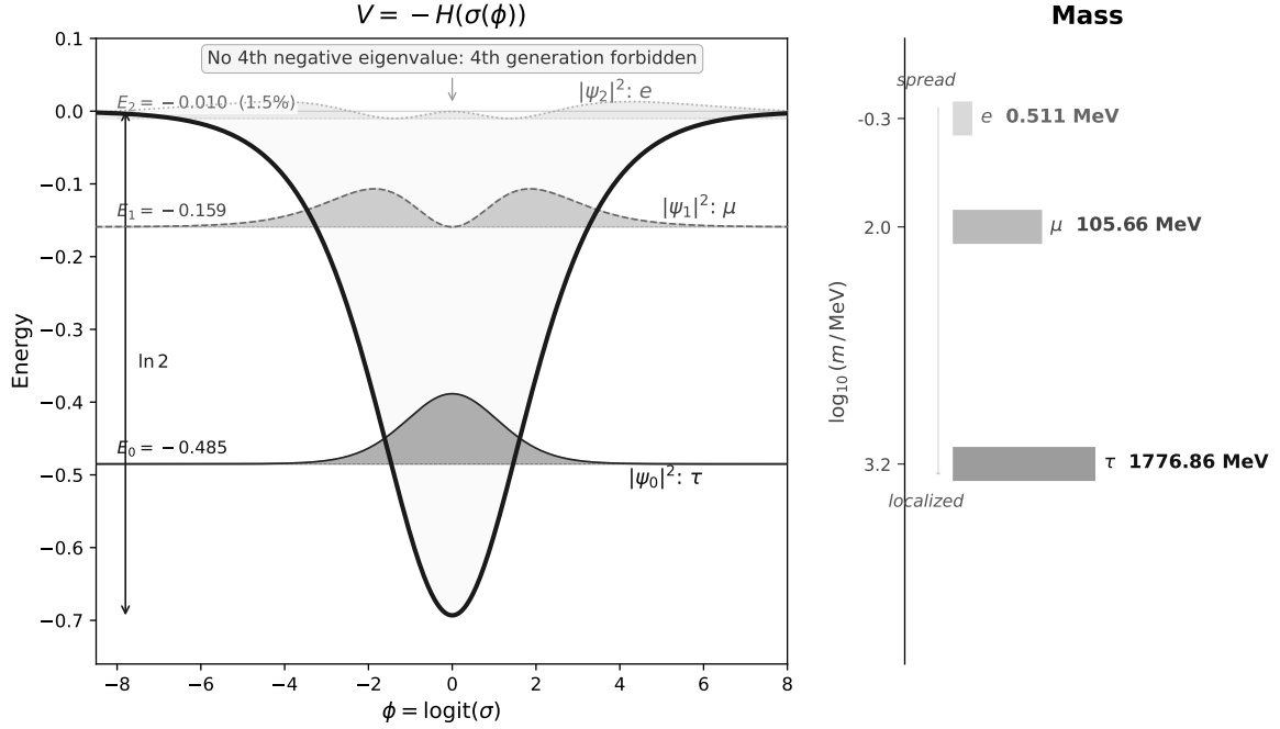
図 1. ポテンシャル V = -H(\sigma(\phi)) とその 3 つの束縛状態の確率密度 |\psi_n|^2 (左)。局在した状態ほど重い粒子に対応する (右)。第 4 の負固有値は存在しない：第 4 世代は存在しない、という予測を与える。
