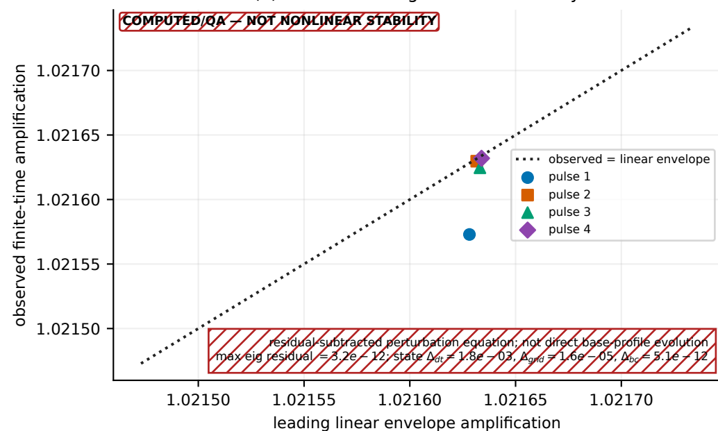
(d) internal leading-mode consistency
