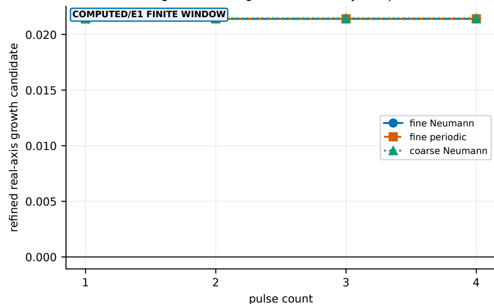
(d) internal leading-mode consistency
