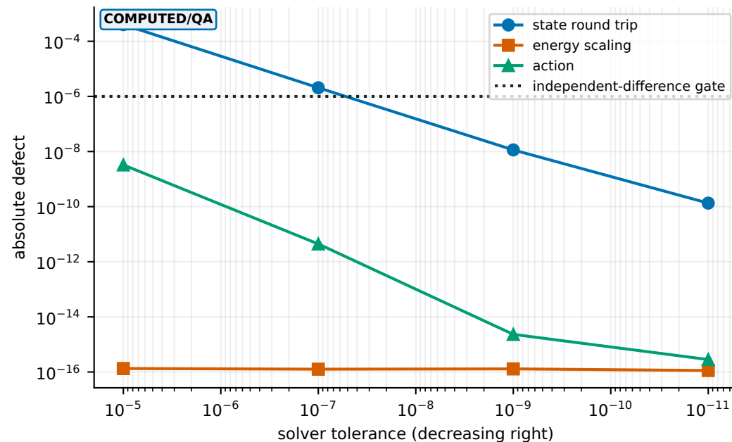
(d) independent physical/central refinement
