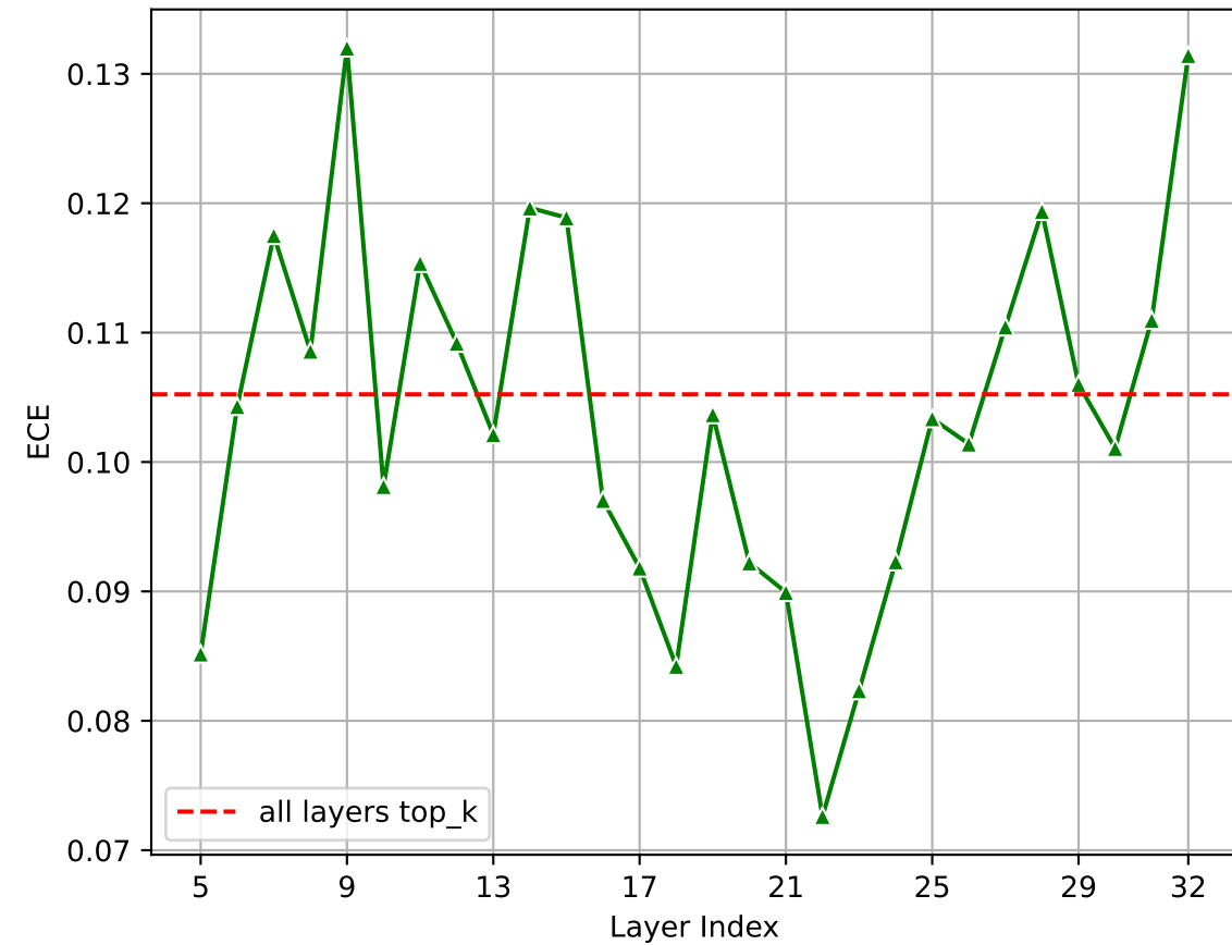
ECE
