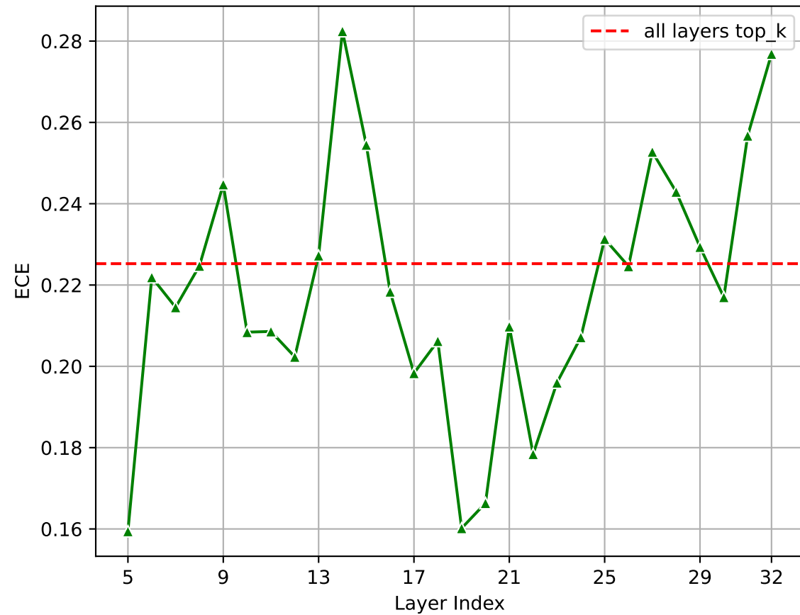
ECE
