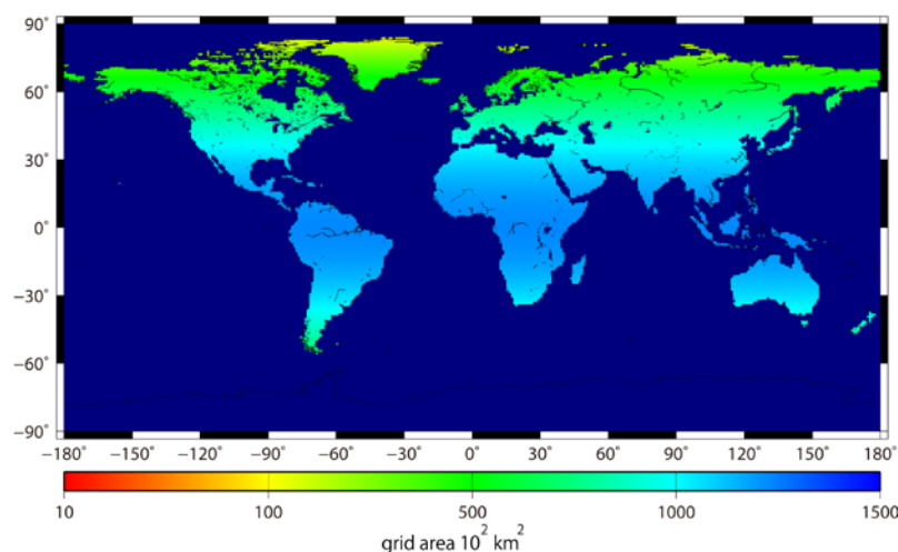
図 6-3 陸域の面積。
