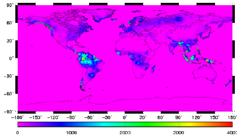
図 8-2 1986 年の年流出量 [mm] 30
