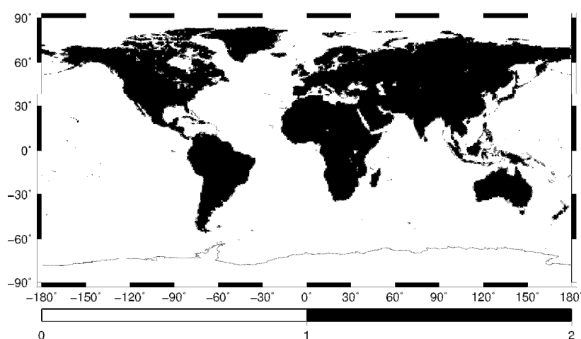
図 6-2 海陸マスク。陸域は 1、海域は 0 を示す。
