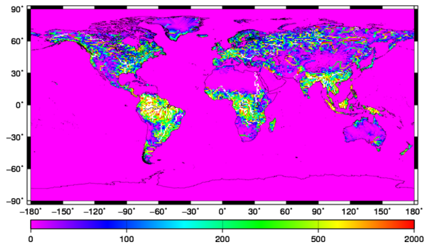
図 9-2 1986 年の年河川流量 [ \text{m}^3 \text{s}^{-1} ]
