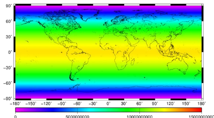
図 6-1 grdara.oneを図化したもの [ \text{m}^2 ]
