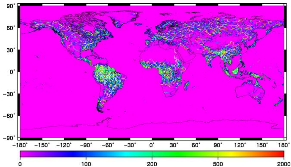
図 9-2 1979 年の年河川流量 [m³ s -1 ]
