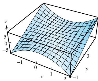
(b) v(x, y) = 3x^2y - y^3
