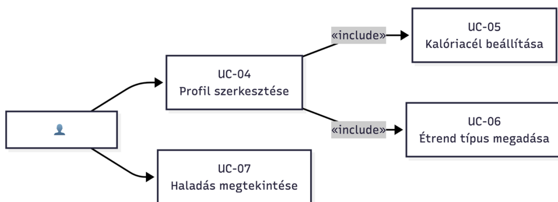
4.1. ábra: Profil beállítás és TDEE-számítás használati eset diagram.
