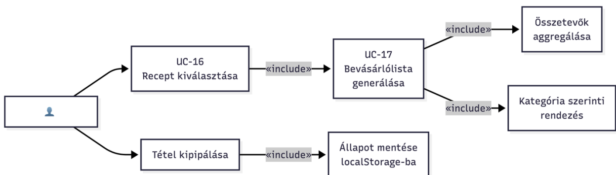
4.4. ábra: Bevásárló lista használati eset diagram
