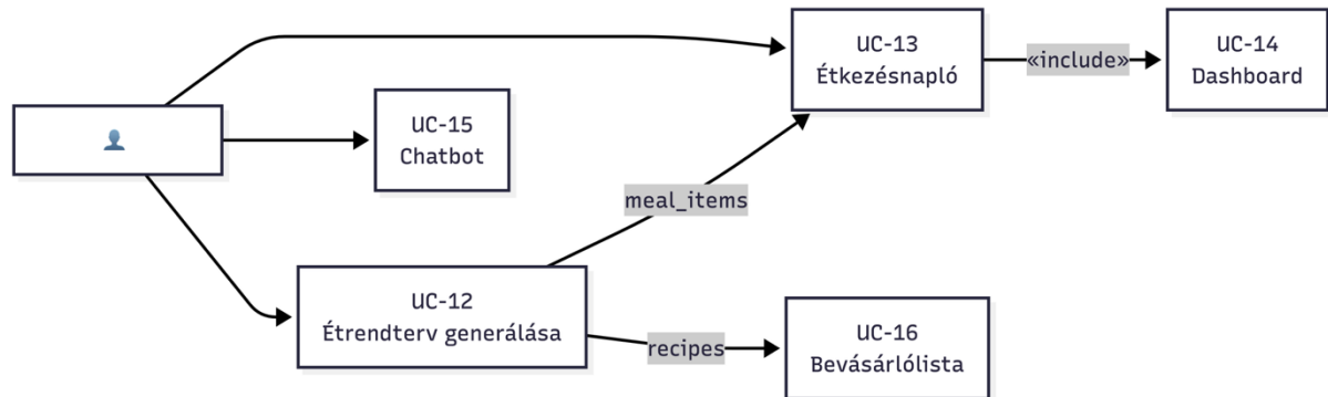
4.3. ábra: Étkezésnapló használati eset diagram
