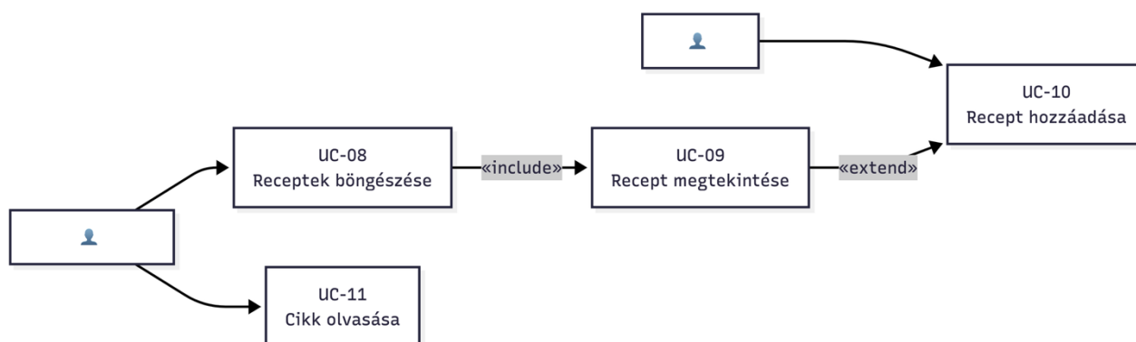
4.2. ábra: Receptkezelés használati eset diagram
