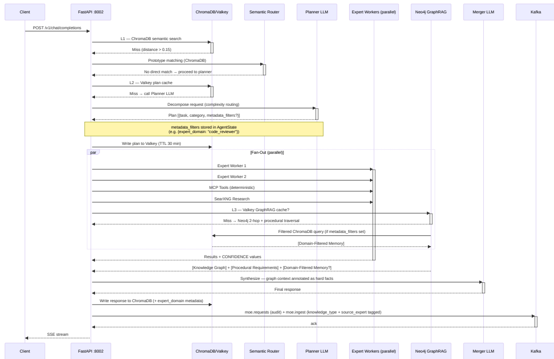
Abbildung 2: End-to-End-Datenfluss einer Chat-Anfrage durch den Orchestrator. Jeder Knoten in der Pipeline ist ein LangGraph-Node mit explizitem Zustand; jeder Kasten ausserhalb der Pipeline ist ein separater Service mit eigener API.
