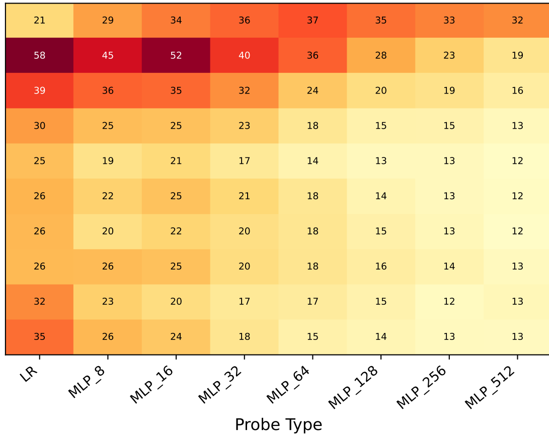
Llama-3
