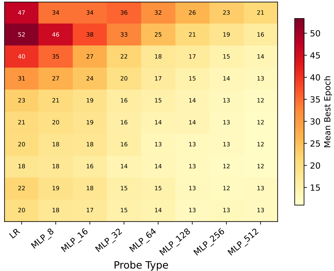
Qwen3
