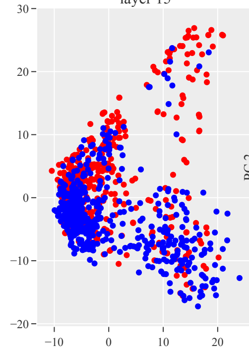
layer 15
