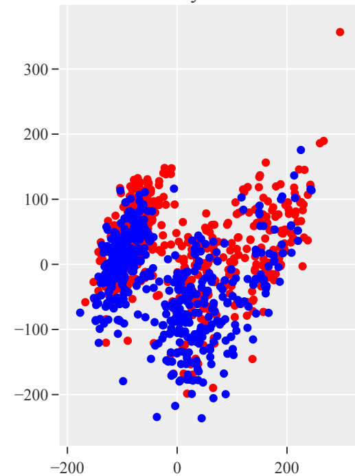
layer 28
