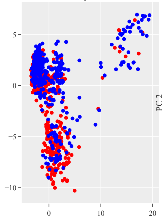
layer 7
