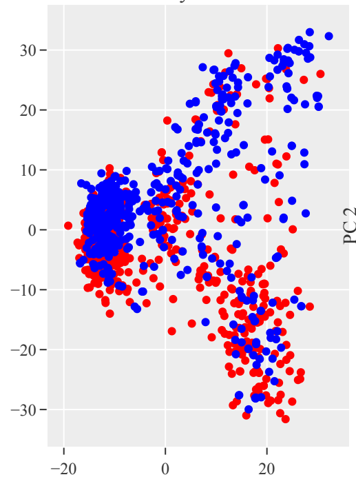
layer 17
