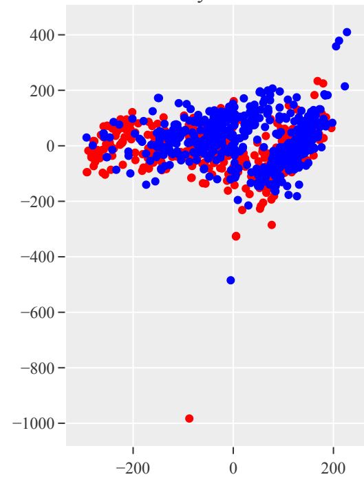
layer 28
