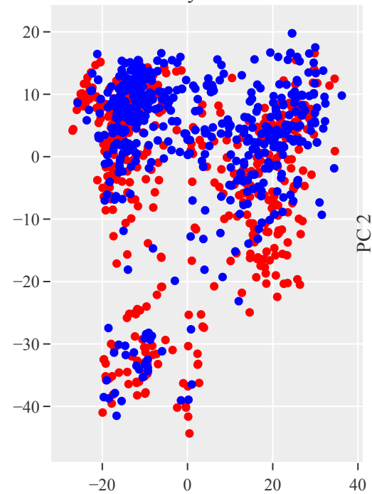
layer 17
