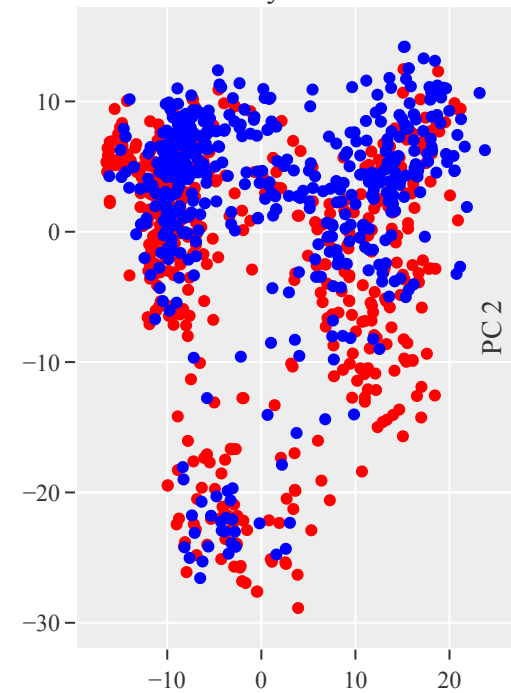
layer 15
