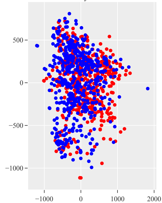
layer 40
