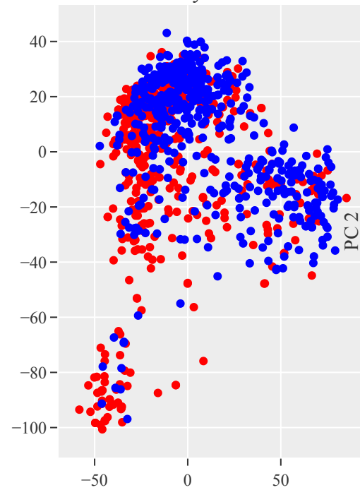
layer 25
