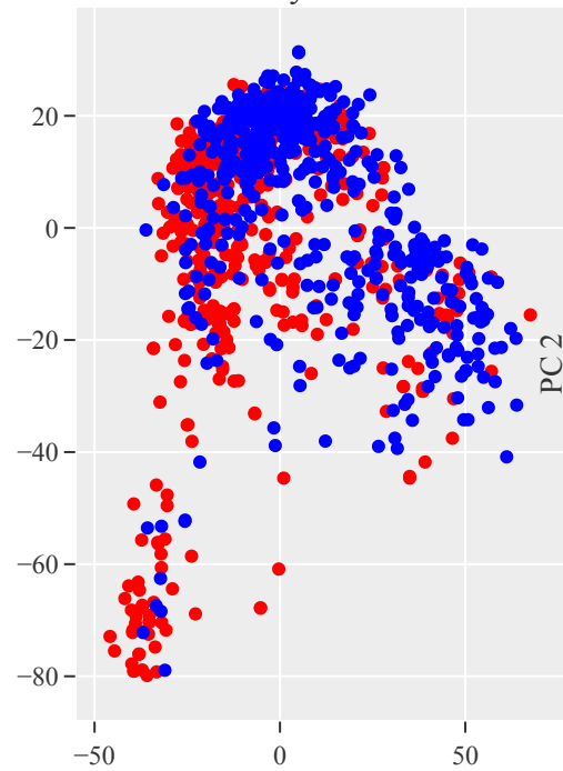
layer 22
