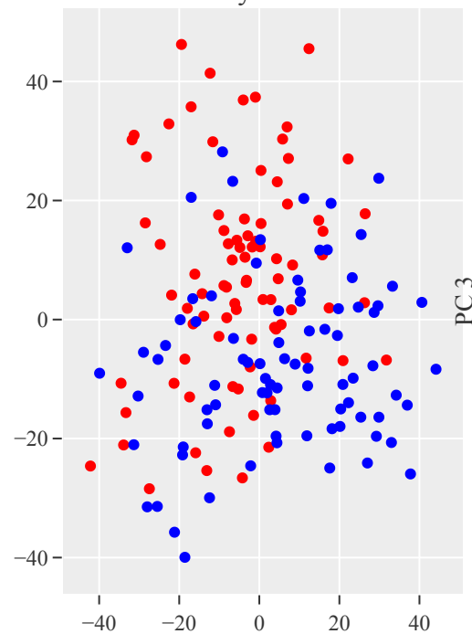
layer 22
