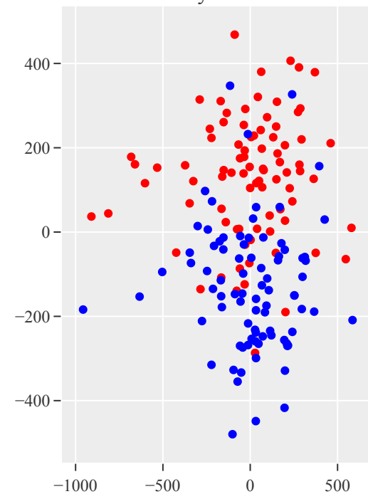
layer 40
