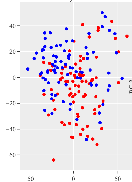
layer 25
