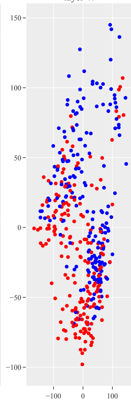
layer 47
