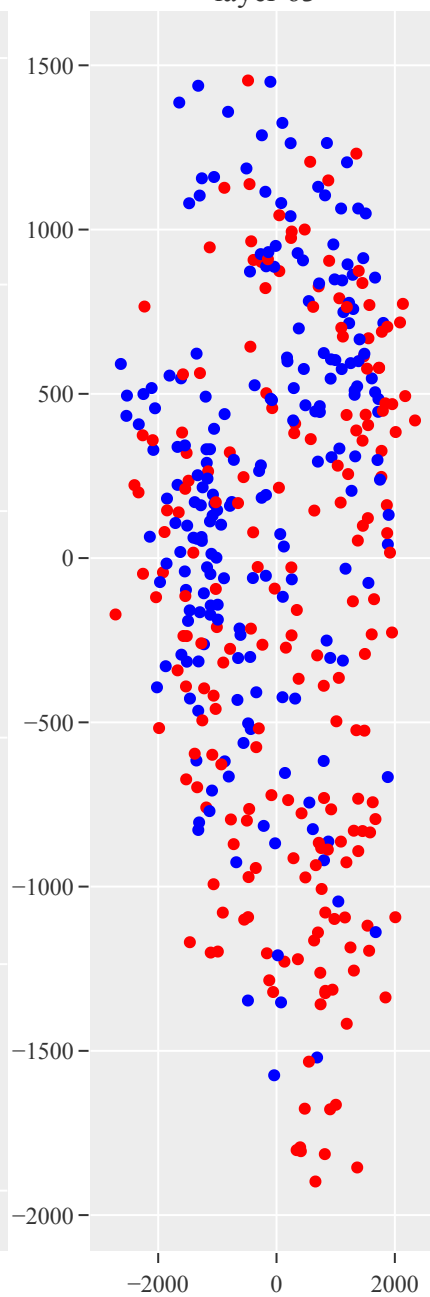
layer 63
