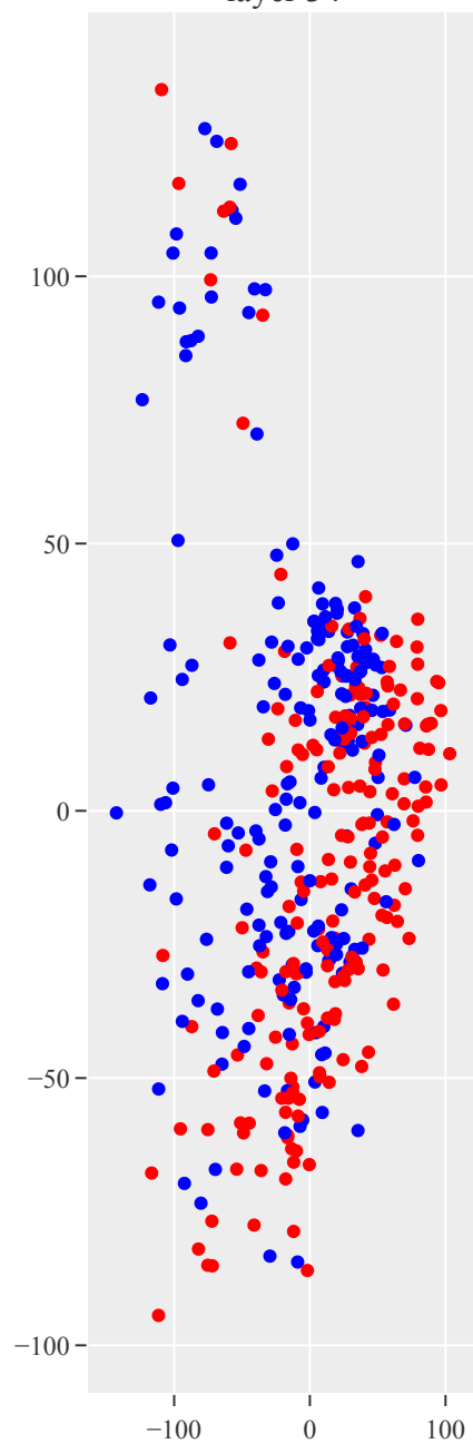
layer 34
