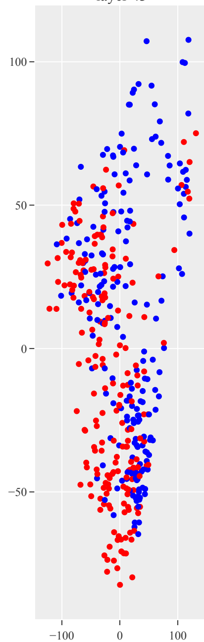
layer 43
