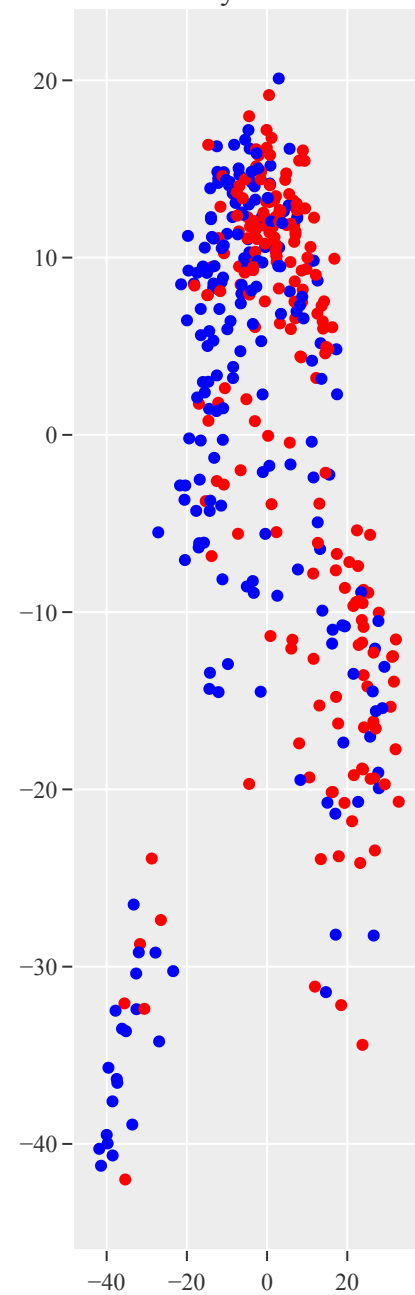
layer 18
