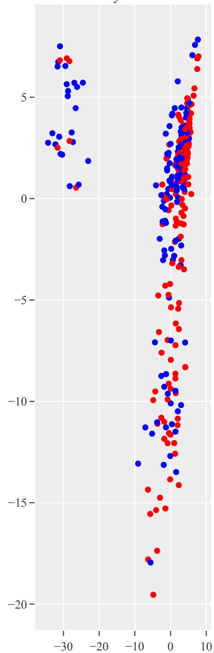
layer 5
