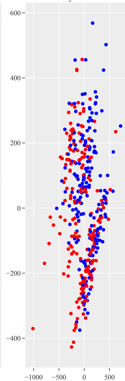
layer 35
