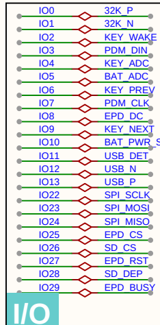
KEY-ADC
