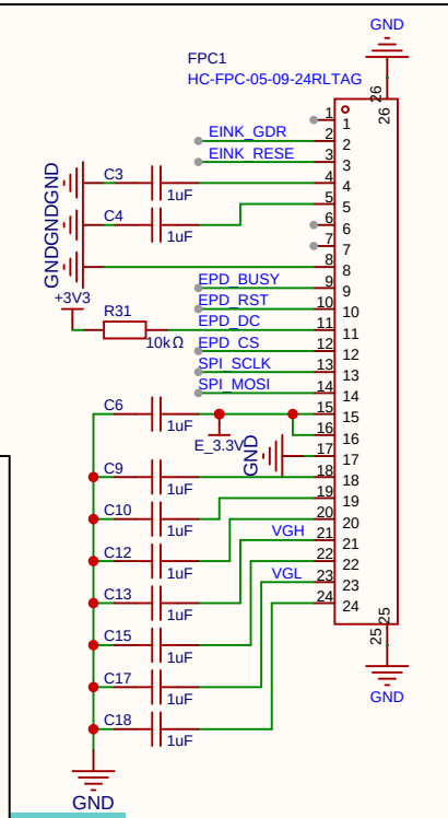
EPD
