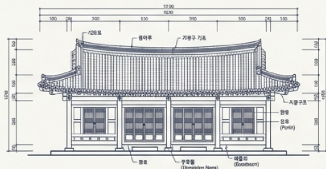
TECHNICAL BLUEPRINT - 한옥 설계도
