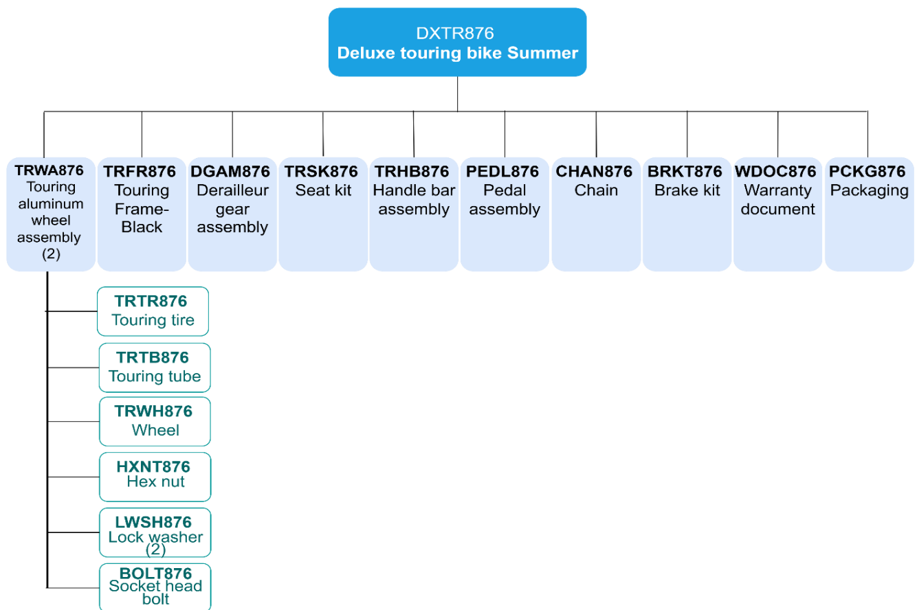
Hình 3.16 BOM của sản phẩm DXTR876 Deluxe touring bike Summer
