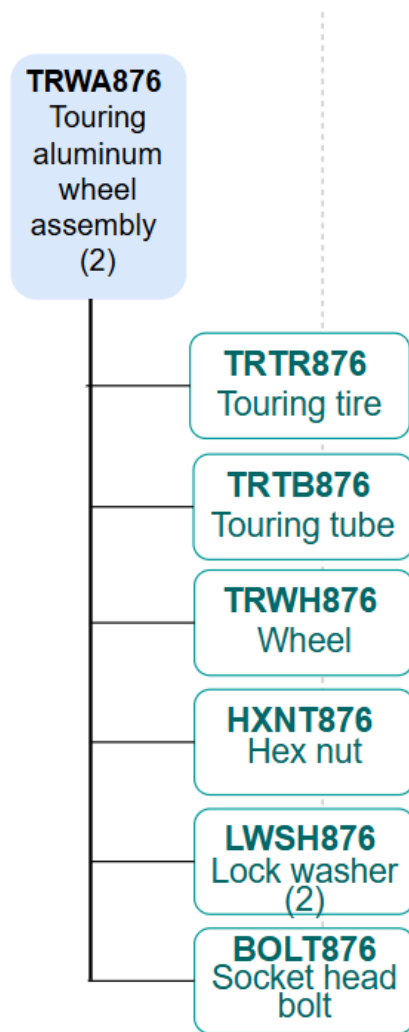
Hình 3.17 BOM của bán thành phẩm TRWA876
