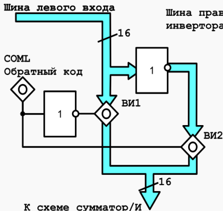
Схема обратного кода
