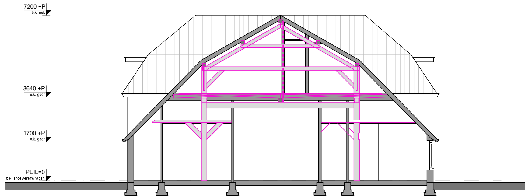
DOORSNEDE A-A
