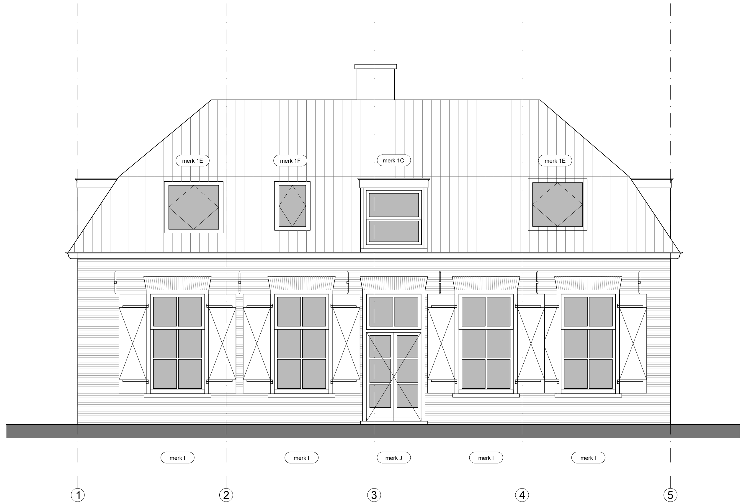
ACHTERGEVEL
