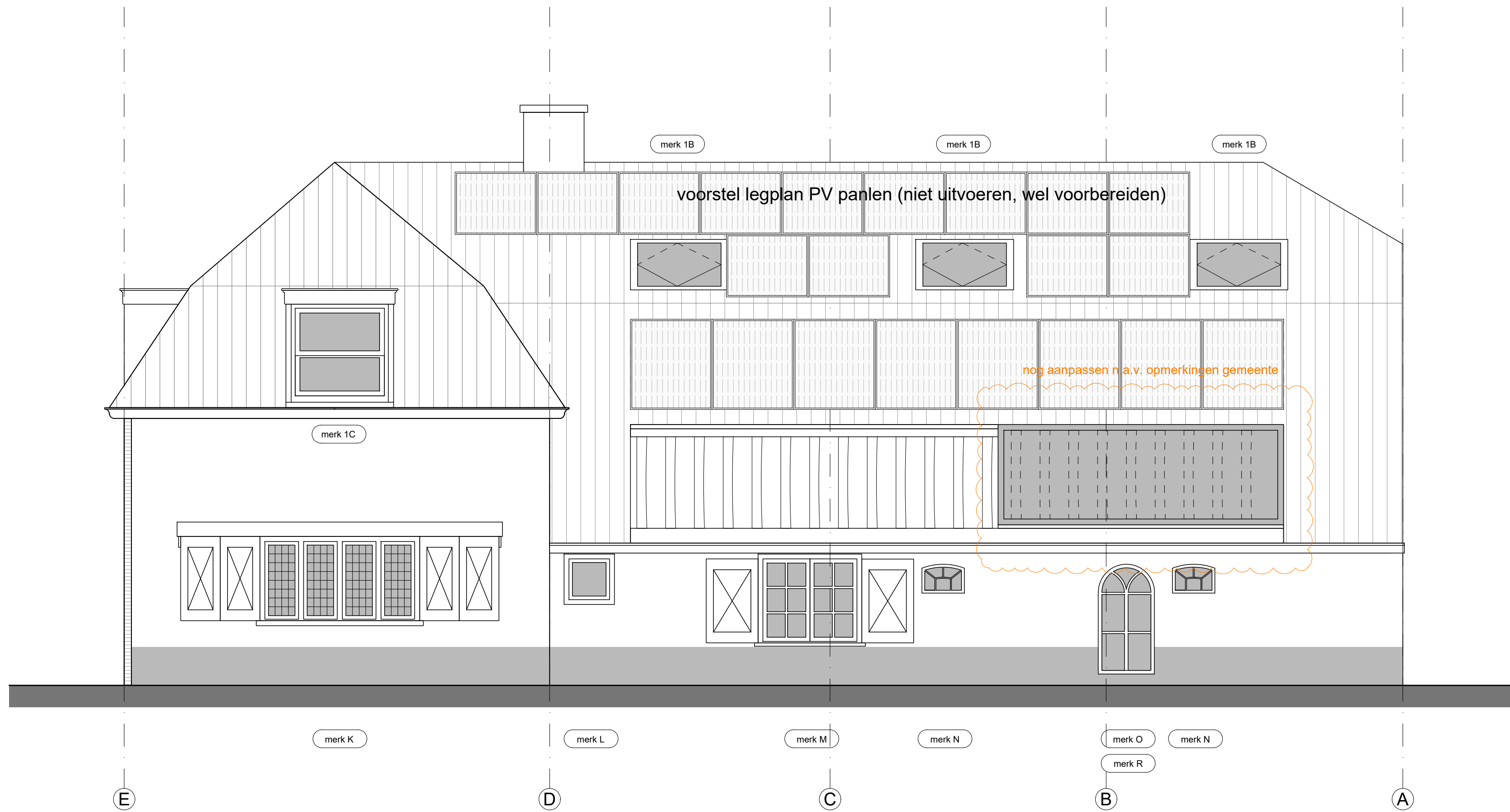
LINKER ZIJGEVEL
