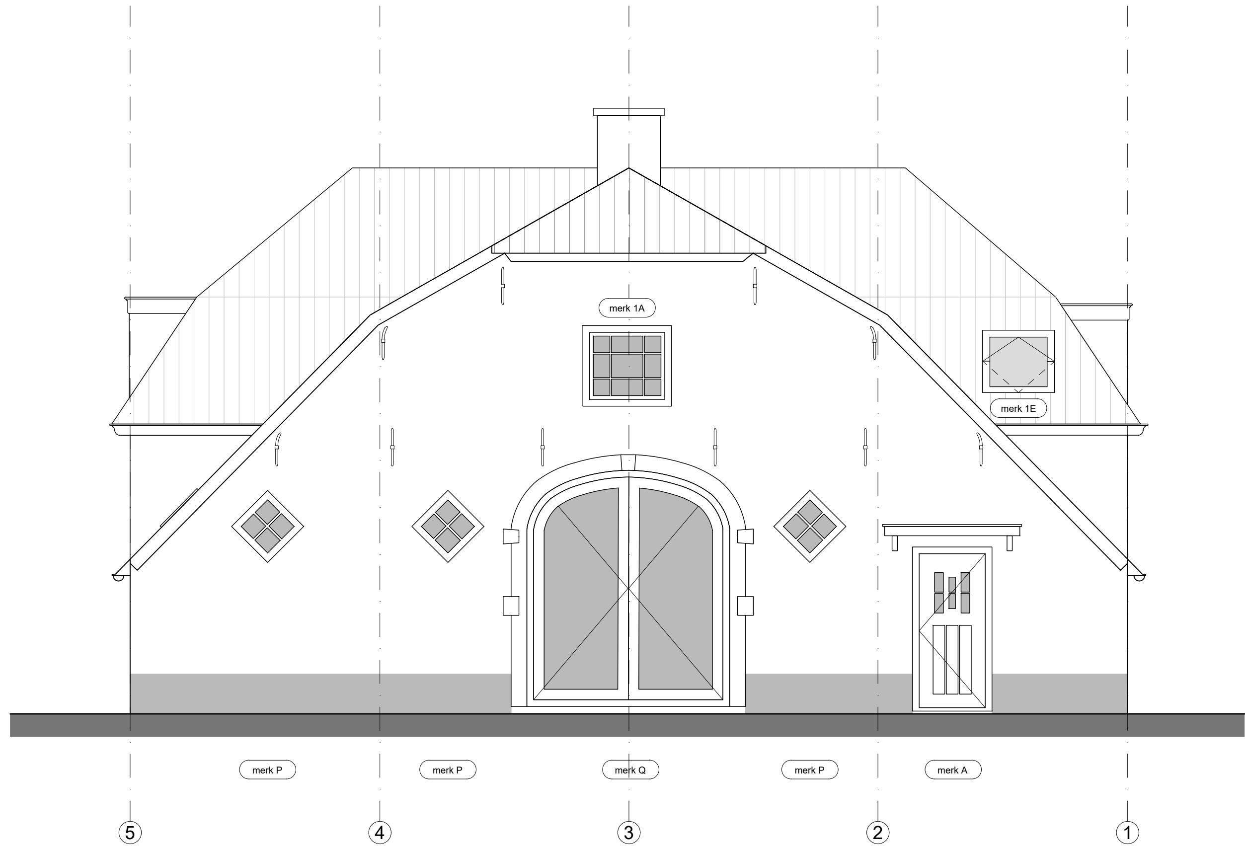
VOORGEVEL
