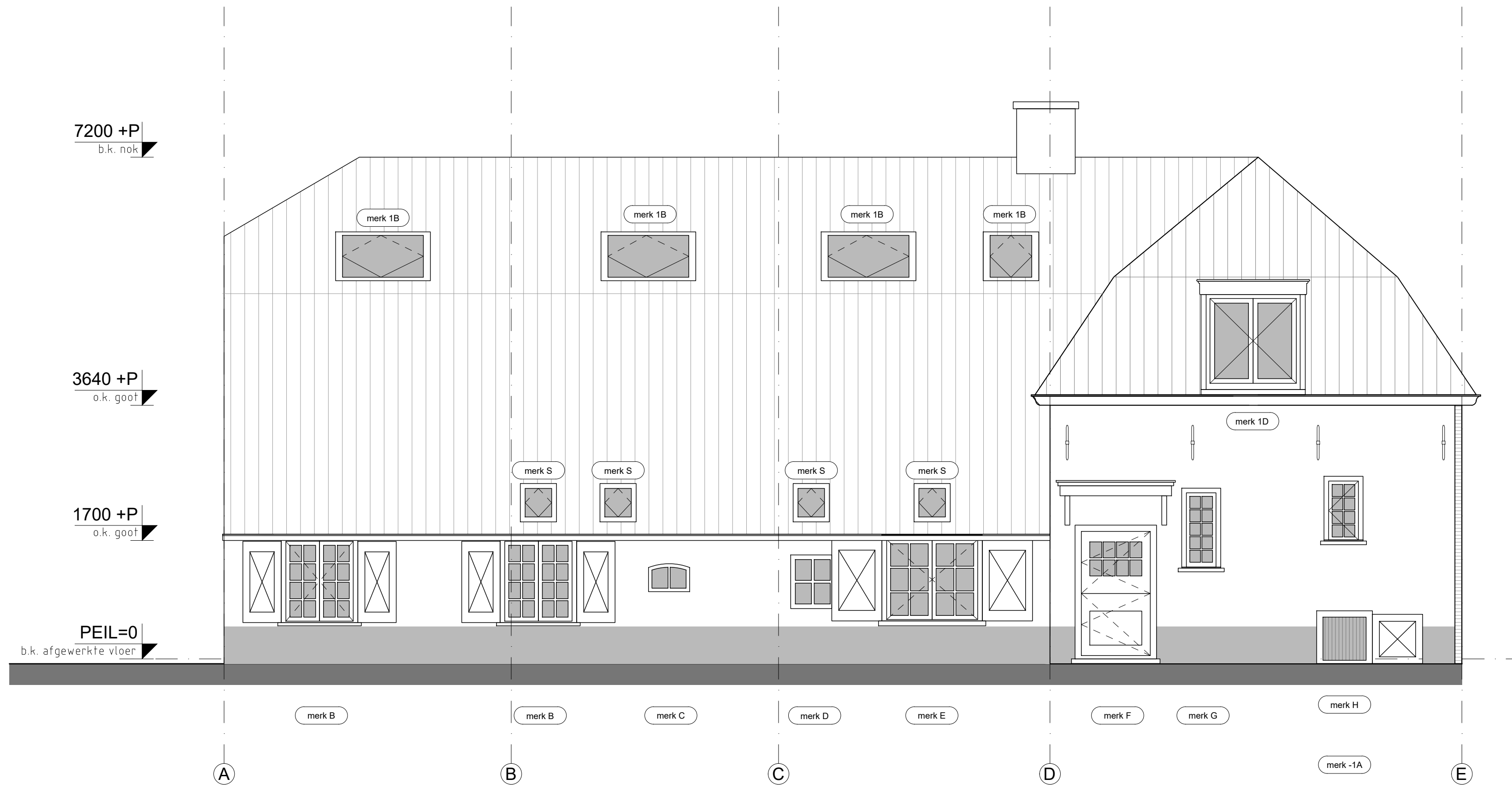
RECHTER ZIJGEVEL
