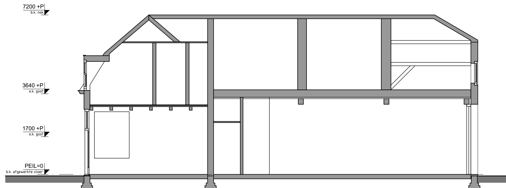
DOORSNEDE B-B
