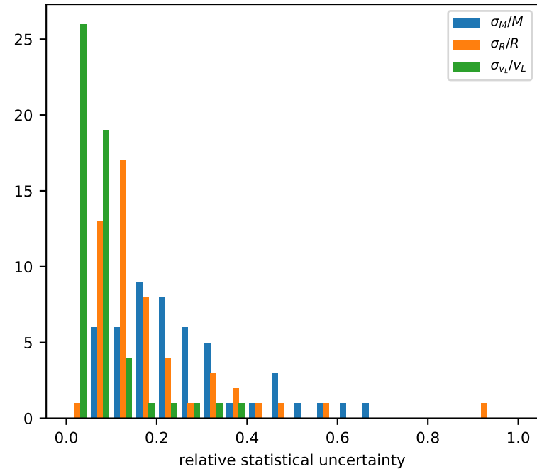
Parameter precision
