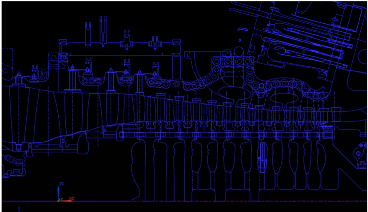
7EA Cross Section
