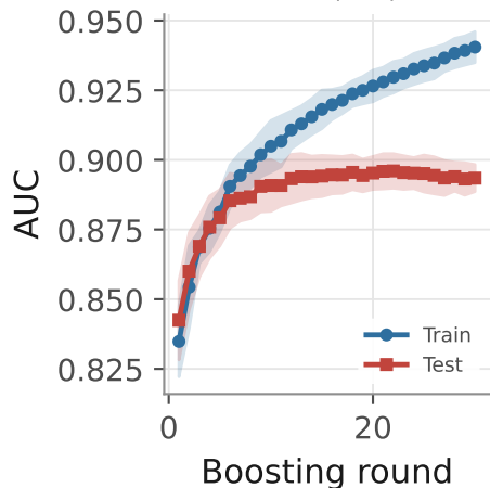
Adult (VFL)
