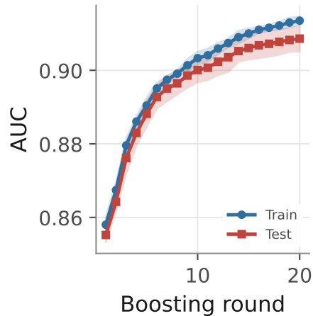
Adult (VFL)
