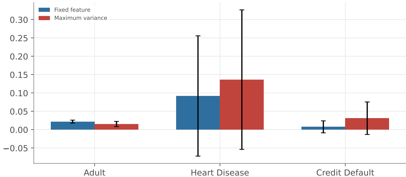
Paired AUC loss (95% CI)
