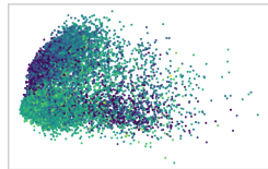
A PCA
