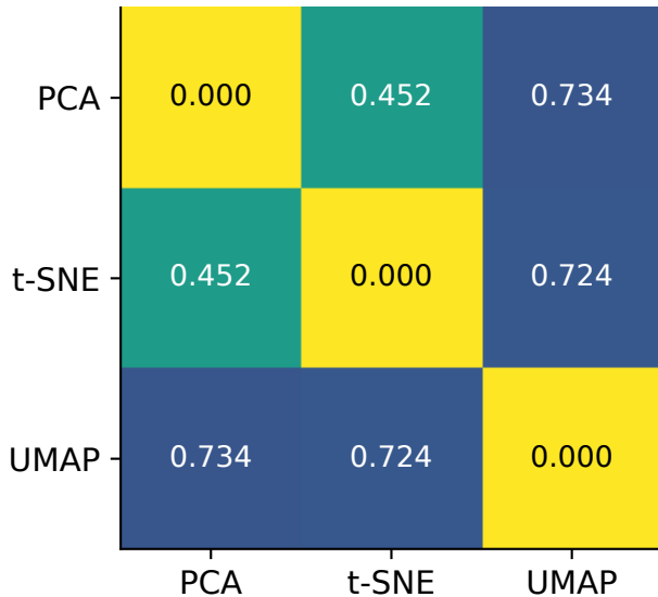
Procrustes disparity
