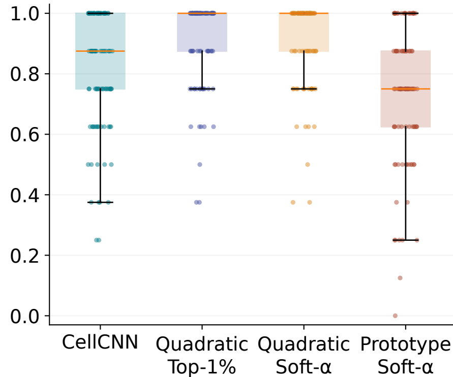
ROC-AUC
