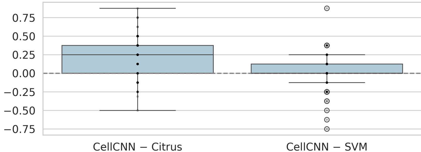
Gepaarte Differenz der ROC-AUC
