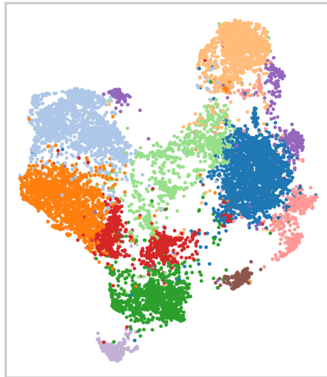
Leiden: 11 Cluster
