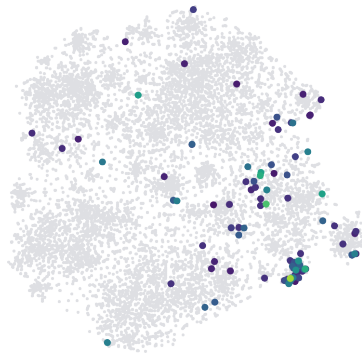
B SVM
