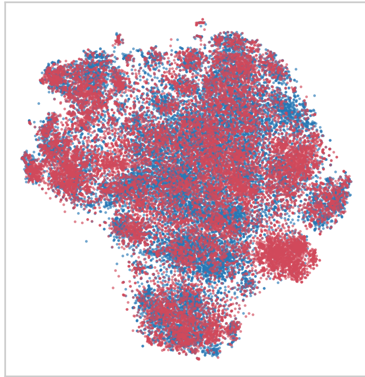
t-SNE
