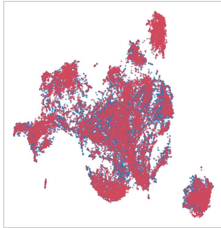
UMAP
