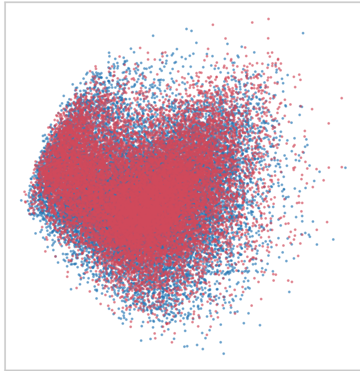
PCA
