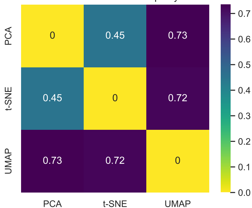
Pairwise Procrustes disparity
