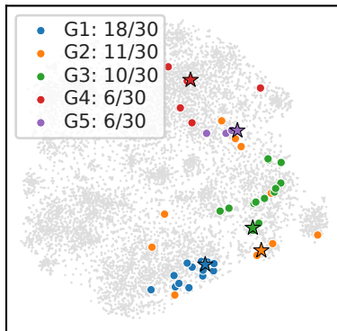
B Citrus-Zentroiden
