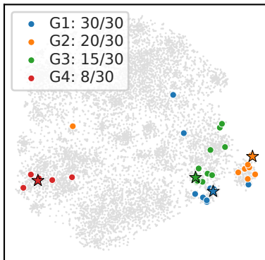
A CellCNN-Zentroiden
