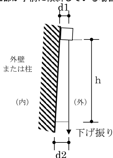
（図１）建物上部が手前に傾斜している場合
