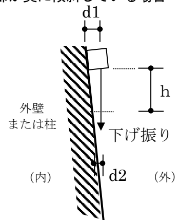
（図２）建物上部が奥に傾斜している場合
