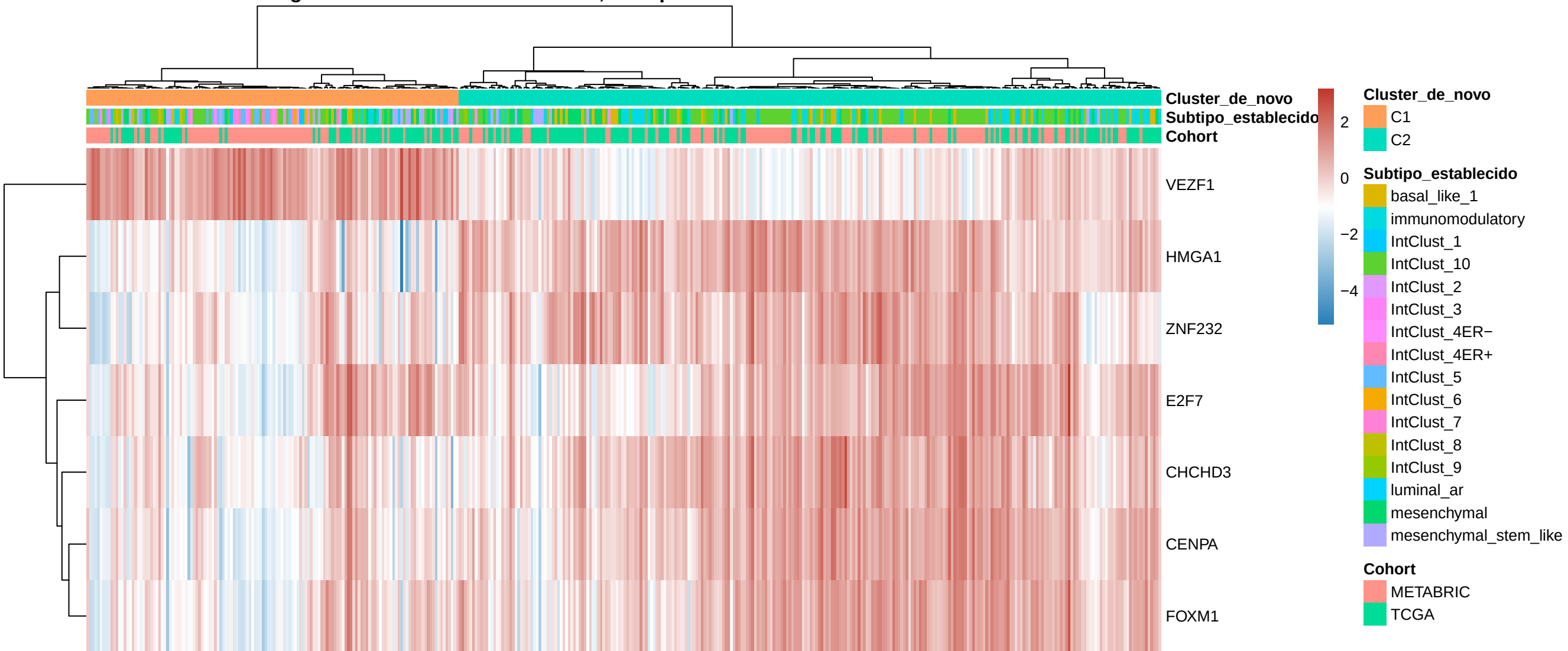
Fig. 1C actualizada – 7 TMR Kbhb, subtipo establecido + cluster de novo
