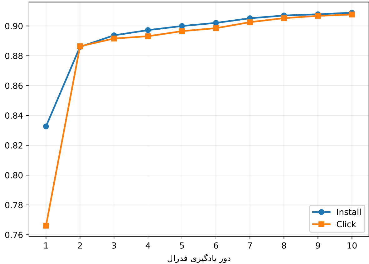
auc
