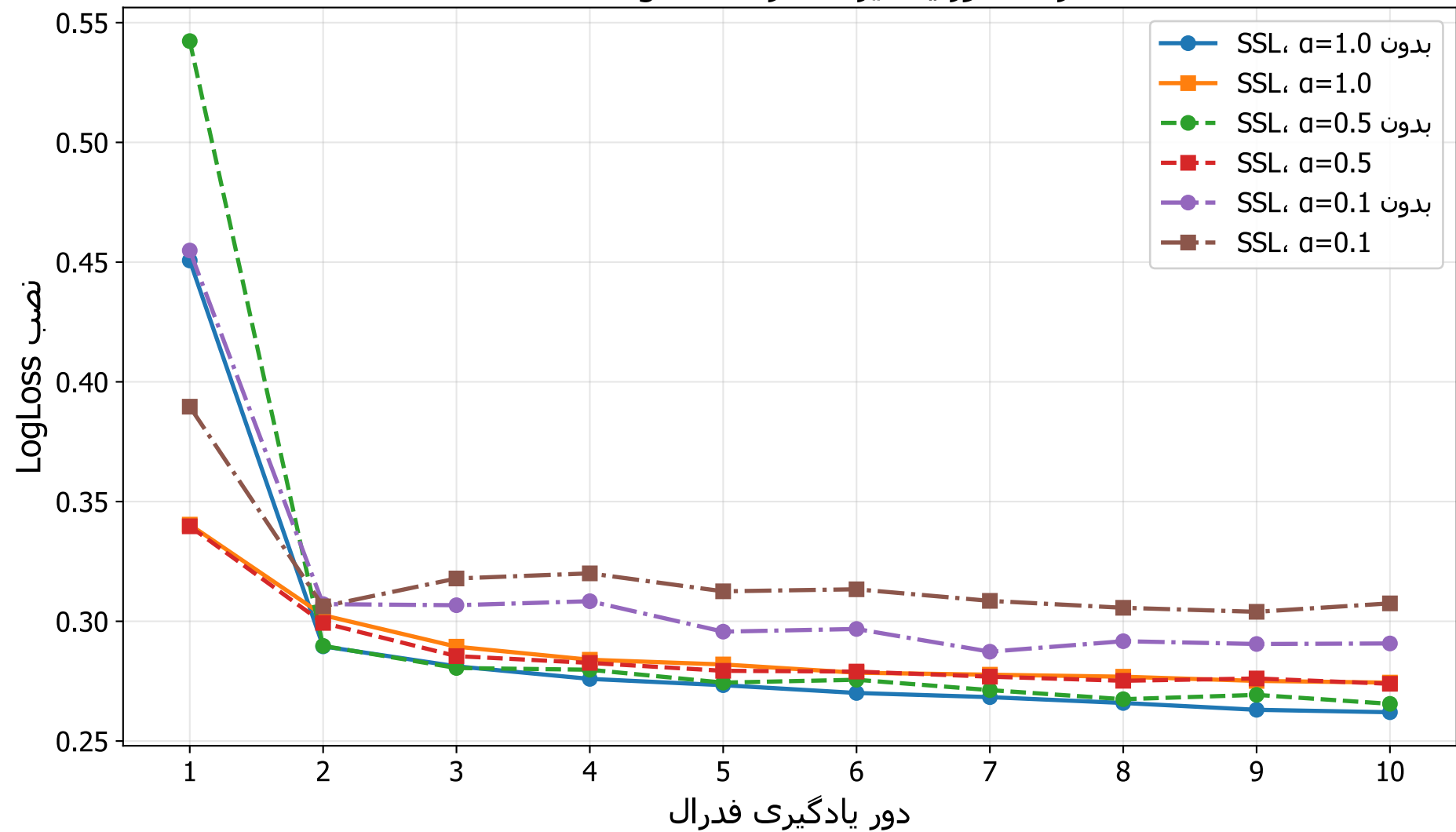
در ۱۰ دور یادگیری فدرال Install LogLoss
