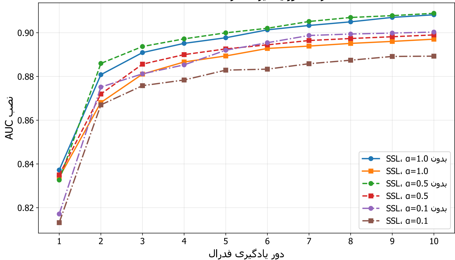
در ۱۰ دور یادگیری فدرال Install AUC
