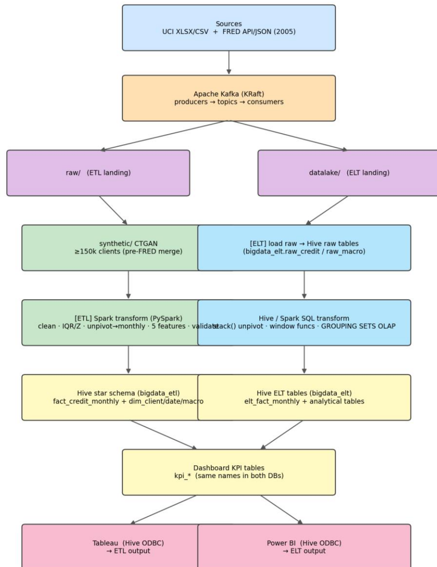
Gambar 3.1 Diagram arsitektur sistem Big Data — jalur ETL dan ELT dari sumber hingga dashboard.
