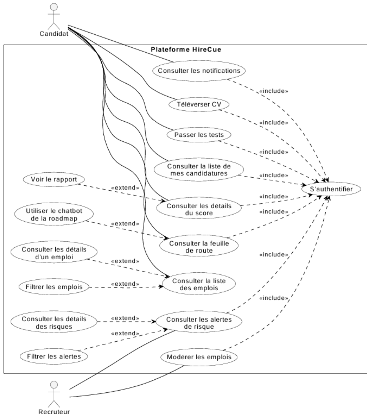
FIGURE 2.6 – Diagramme de cas d'utilisation global de la plateforme HireCue
