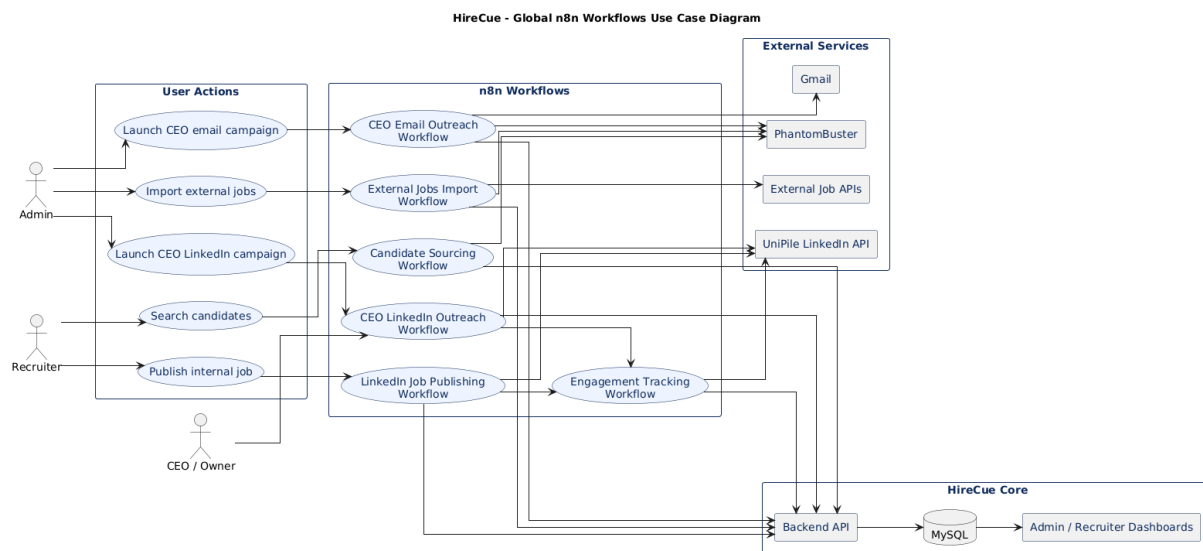
FIGURE 2.8 – Diagramme de cas d'utilisation global des workflows n8n de HireCue
