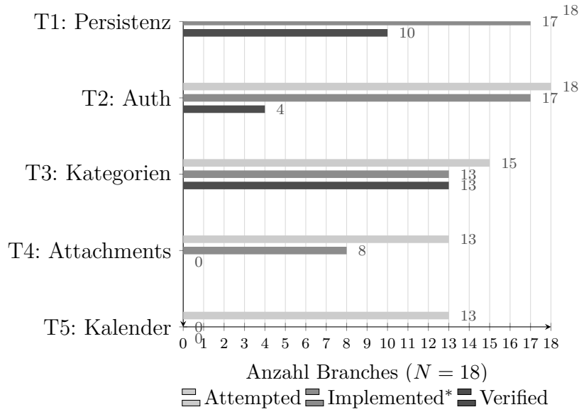
Abbildung 6.1: Pipeline-Ergebnisse für T1–T5 ( N = 18 ) als gruppierte Balken: Attempted (Chat-Signal), Implemented* (definiert als Attempted \wedge (Implemented_{static} \vee Verified) ) und Verified (testgebunden: bestandene V3-Integrationstests). Die Werte entsprechen Tabelle 6.2.
